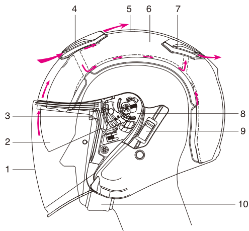
Σύστημα εξαερισμού κατά της θάμβωσης της ζελατίνας System wentylacji zapobiegający zaparowaniu osłony
