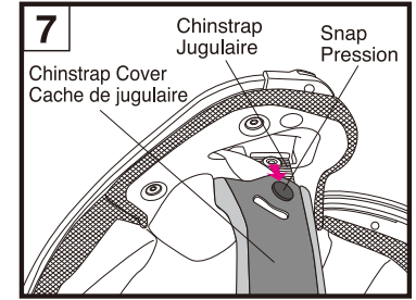
Chinstrap Cover (R) Chinstrap Cover (L) Cache de jugulaire (droit) Cache de jugulaire (gauche)
