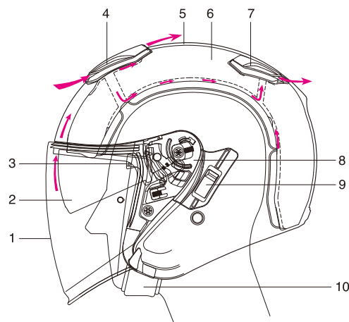
Visier Antibeslags Ventilations System Sistema di ventilazione visiera anti-condensa
